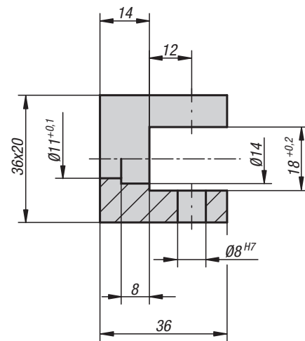
clevis
